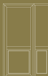
Porte E1 avec tierce fixe et soubassement platebande
