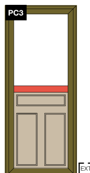
Panneau double forme cimaise filante
