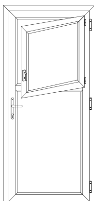
PORTE PAYSANNE (ouvrant dans l'ouvrant)
